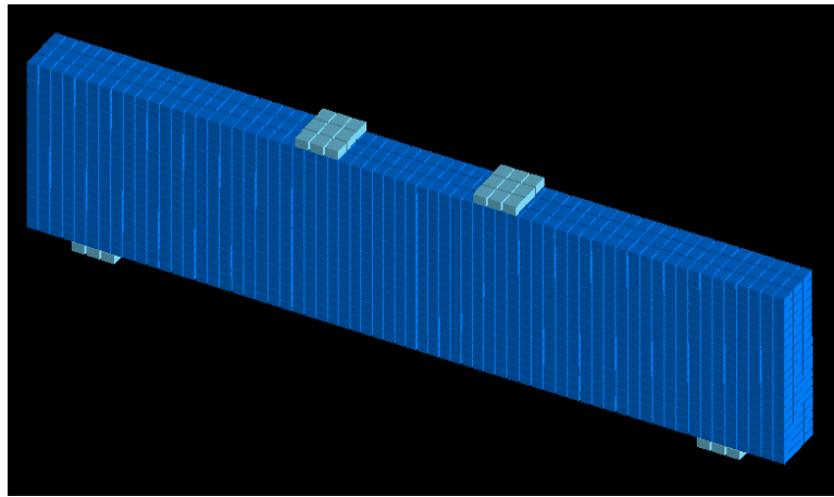
Fig. 1.b ELS mesh.
