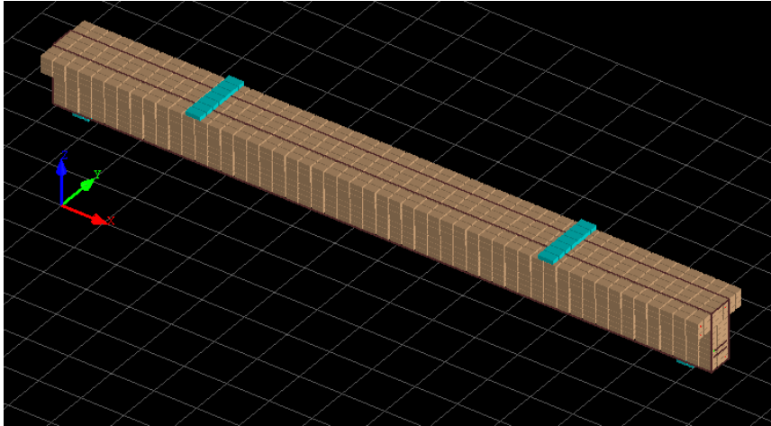
Fig. 1.b ELS mesh
