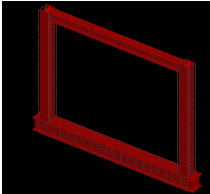
Fig. 1.b ELS mesh.
